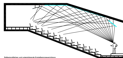
Reflexionsflächen und unterstützende Erstreflexionsausrichtung
