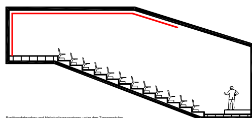
Breitbandabsorber und Helmholtzresonatoren unter den Treppenstufen
