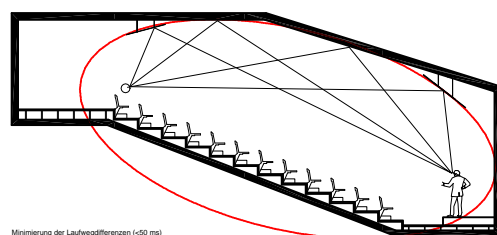
Minimierung der Laufwegdifferenzen (<math>< 50 \text{ ms}</math>)
