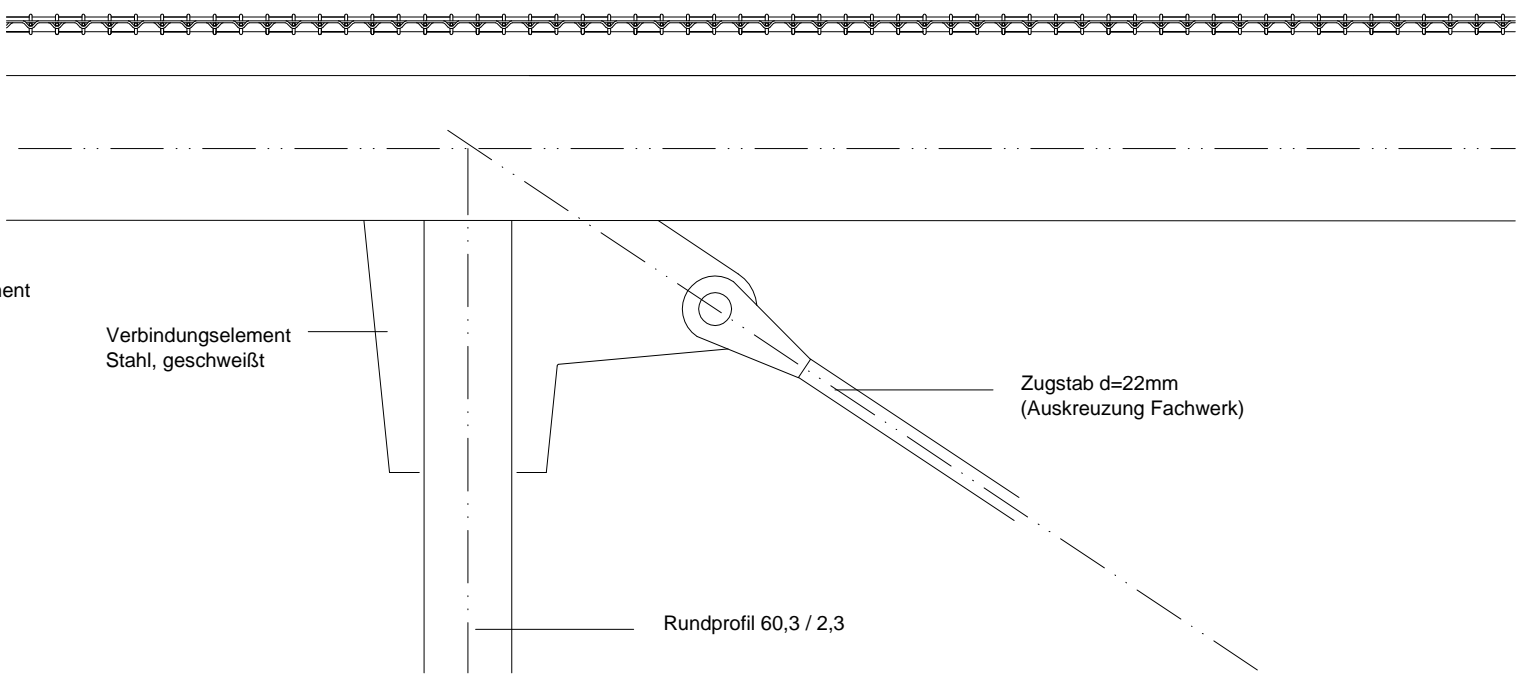
Pos.1.2 - Knotenpunkt
