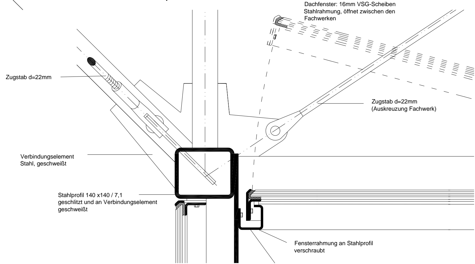
Pos.1.5 - Knotenpunkt
