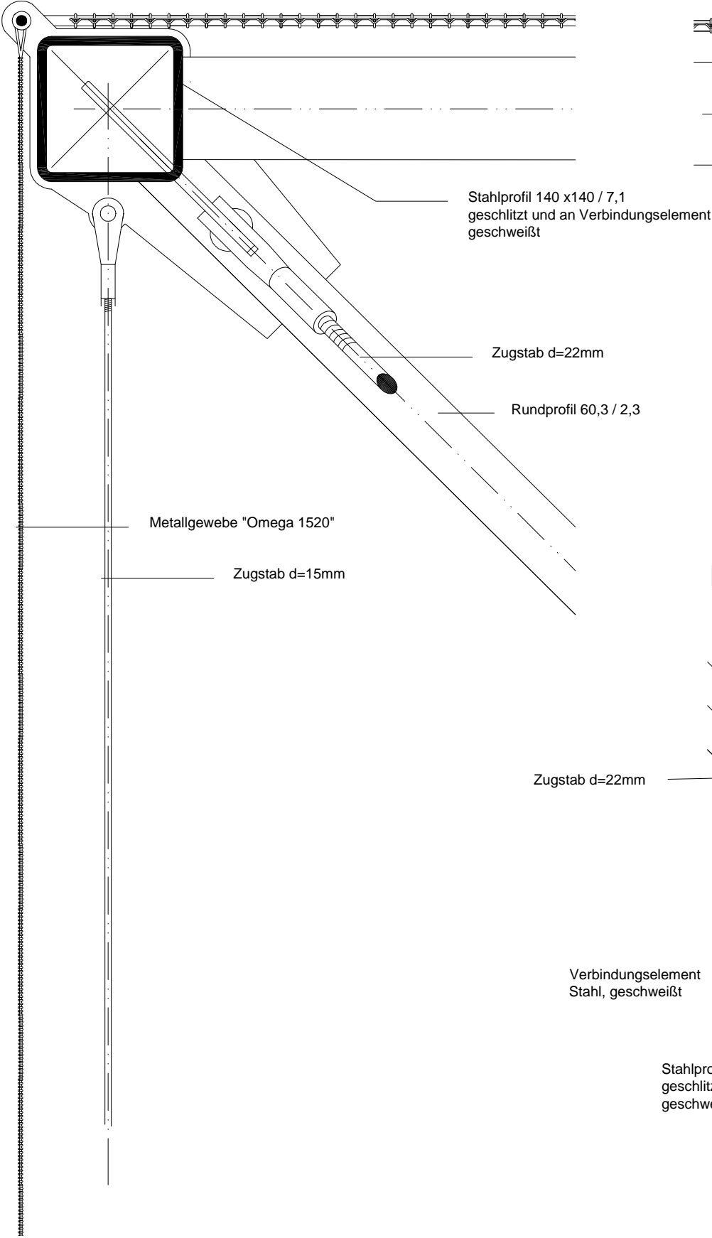
Pos.1.1 - Knotenpunkt
